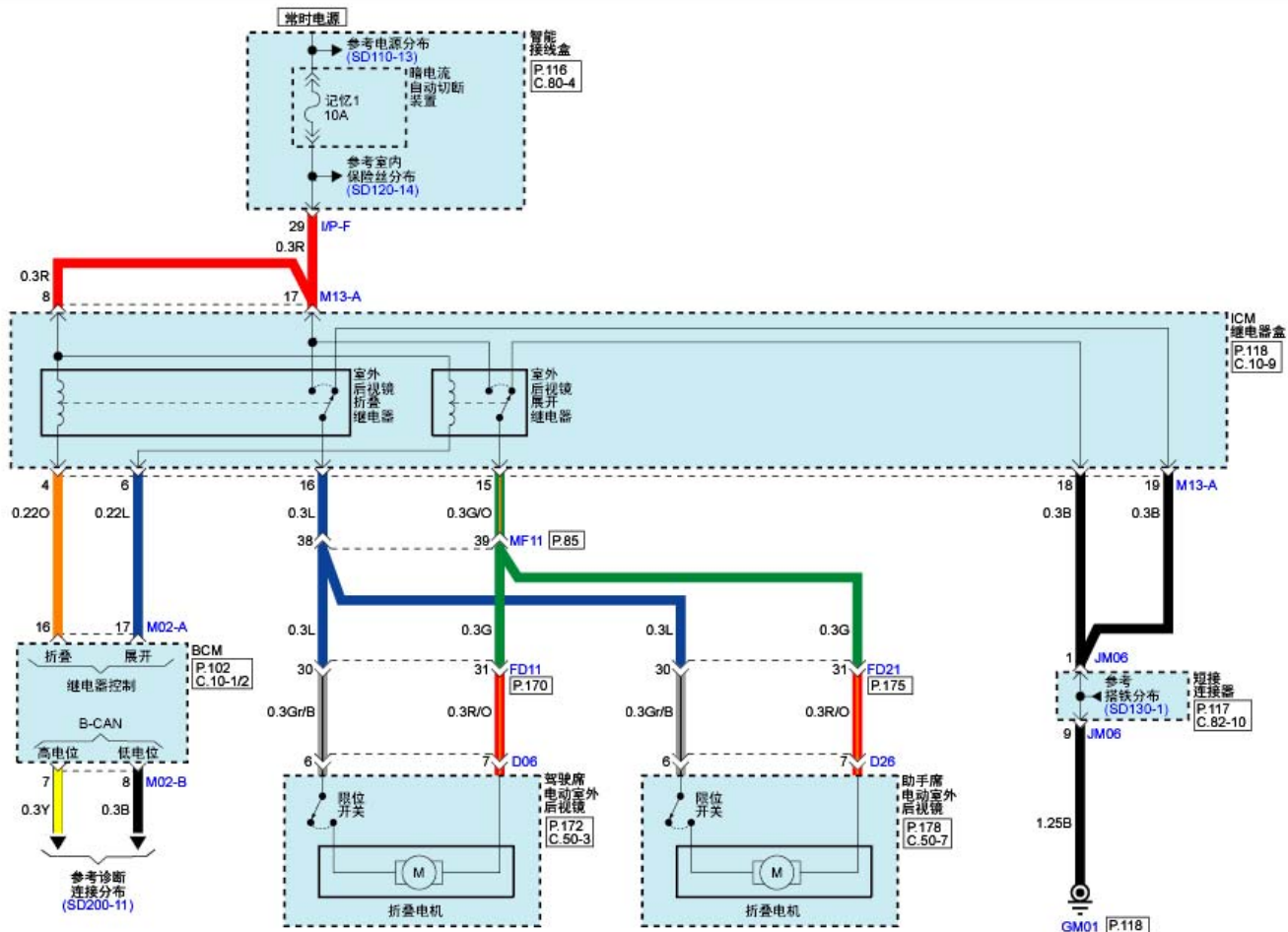
室外后视镜折叠系统(1)
